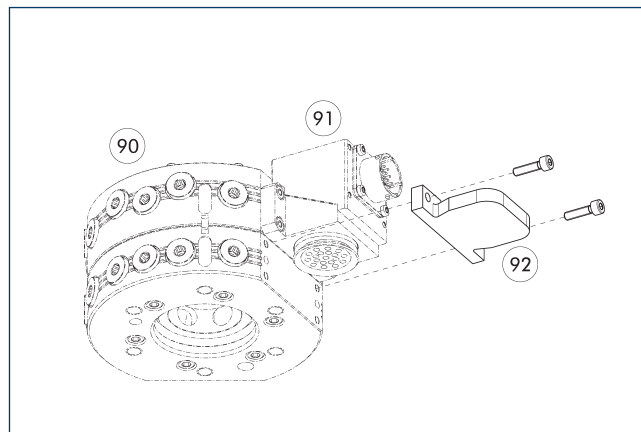
90 Changeurs d'outils automatisés CPS
